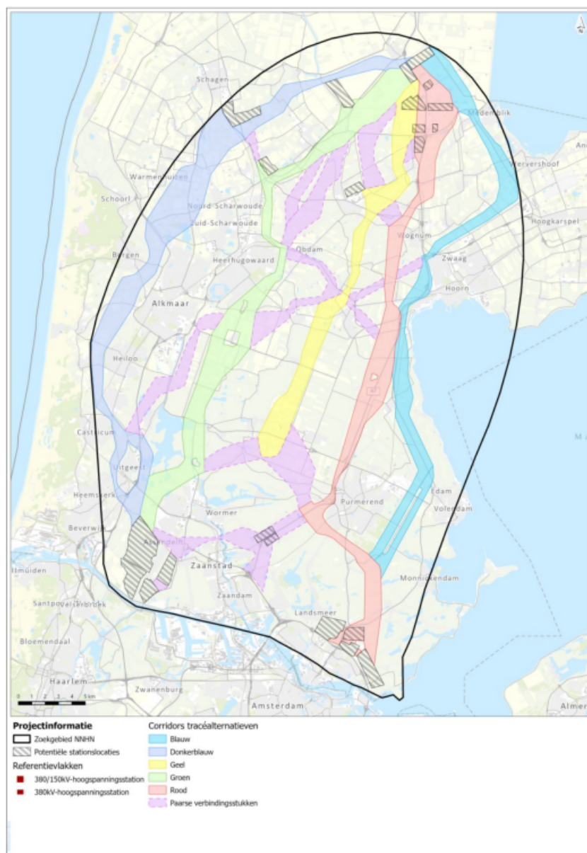
Figuur 3.2 Onderzoeksalternatieven 380 kV-Netuitbreiding Noord-Holland Noord
